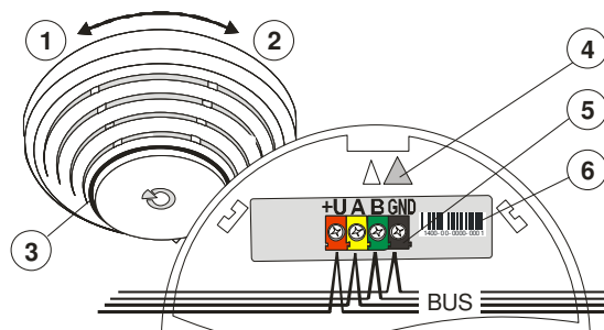
Rys 6: 1 - otwieranie (zdejmovanie) obudowy czujnika; 2 - zamykanie (zakładanie) obudowy czujnika; 3 - czujnik optyczny; 4 - strzałka wskazująca miejsce wstawienia czujnika; 5 - złącza magistrali 6 - kod produkcji
